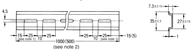
DIN Track PFP-100N2
